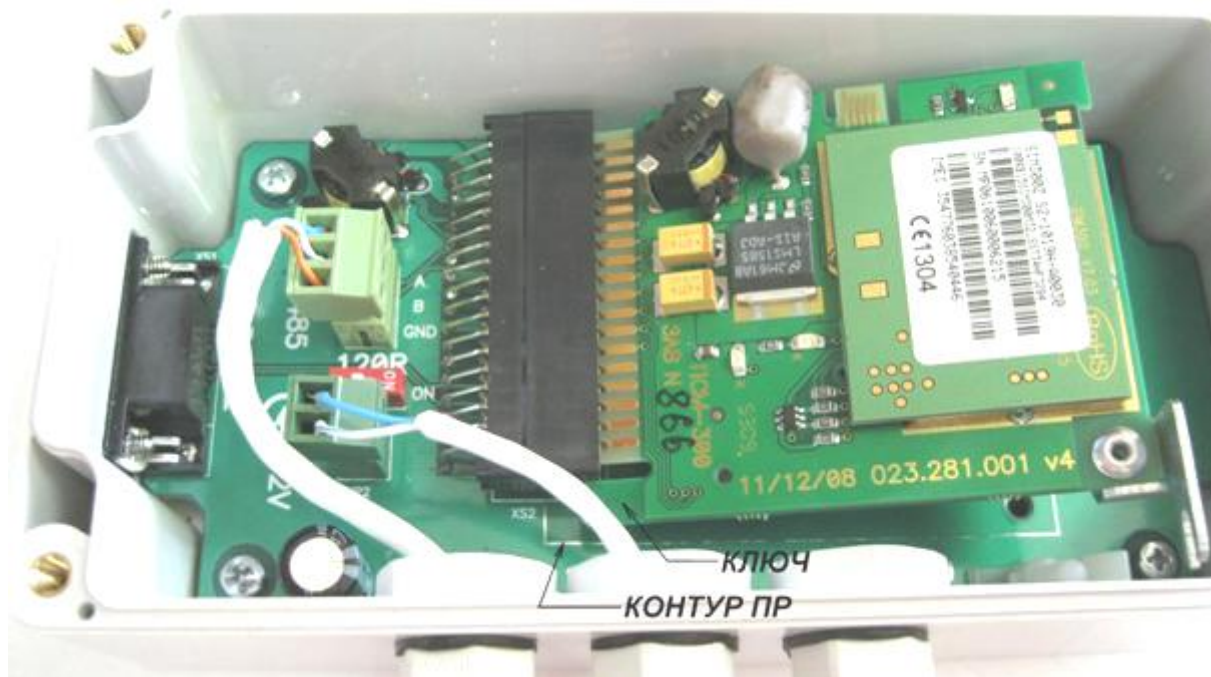
Рисунок 17.8. Установка ПР теплосчетчика МКТС в УППР.
