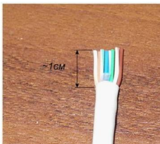
Рисунок 12.3 Удаление излишков проводников
