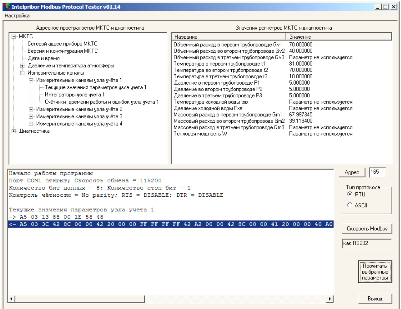
Рисунок 4.12 Просмотр выбранной области памяти МКТС.
