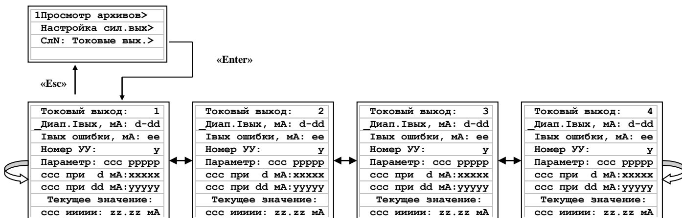
Рисунок 7.4 Схема меню токовых выходов МКТС
