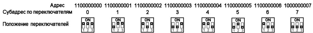
Рисунок 13.3 Установка адреса П4Р строенным переключателем
