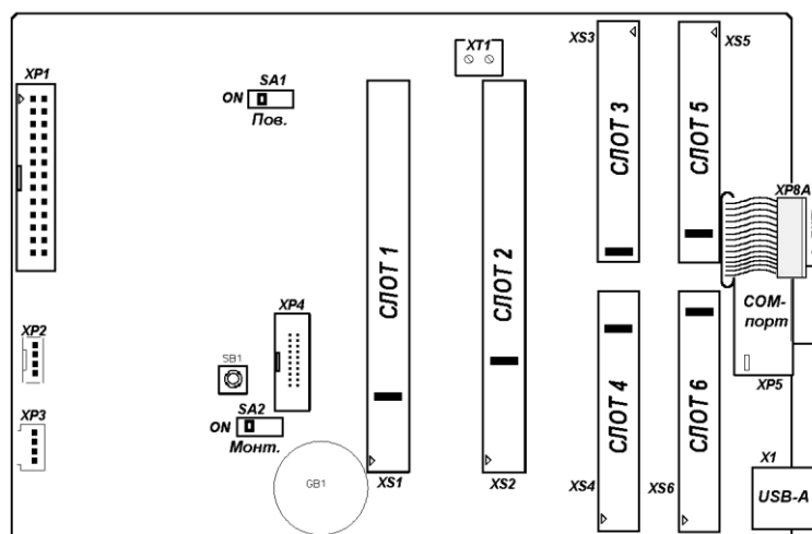
Рисунок 14.4 Материнская плата СБ МКТС (СБ-Т20*4 и СБ-02)
