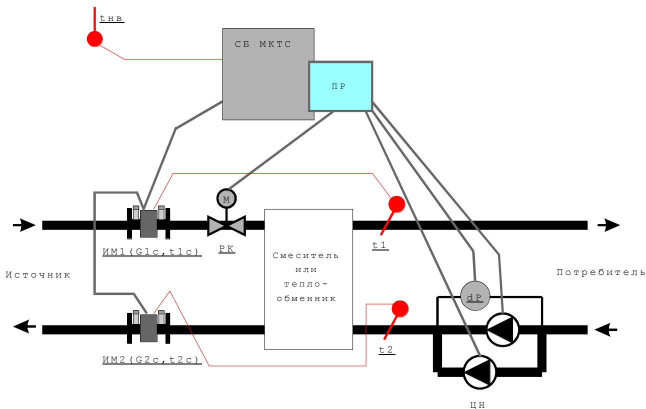
Рисунок 10.1. Схема применения платы регулирования.
