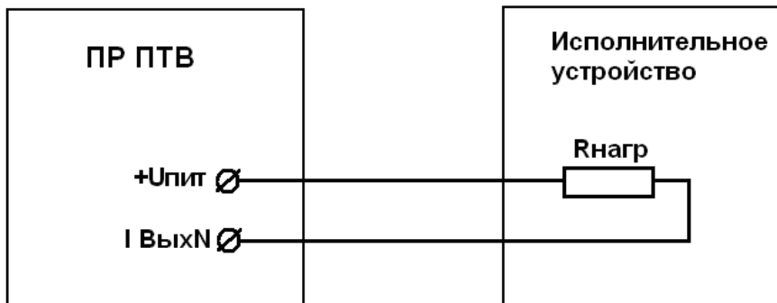
Рисунок 7.2 Подключение исполнительного устройства к токовому выходу.
