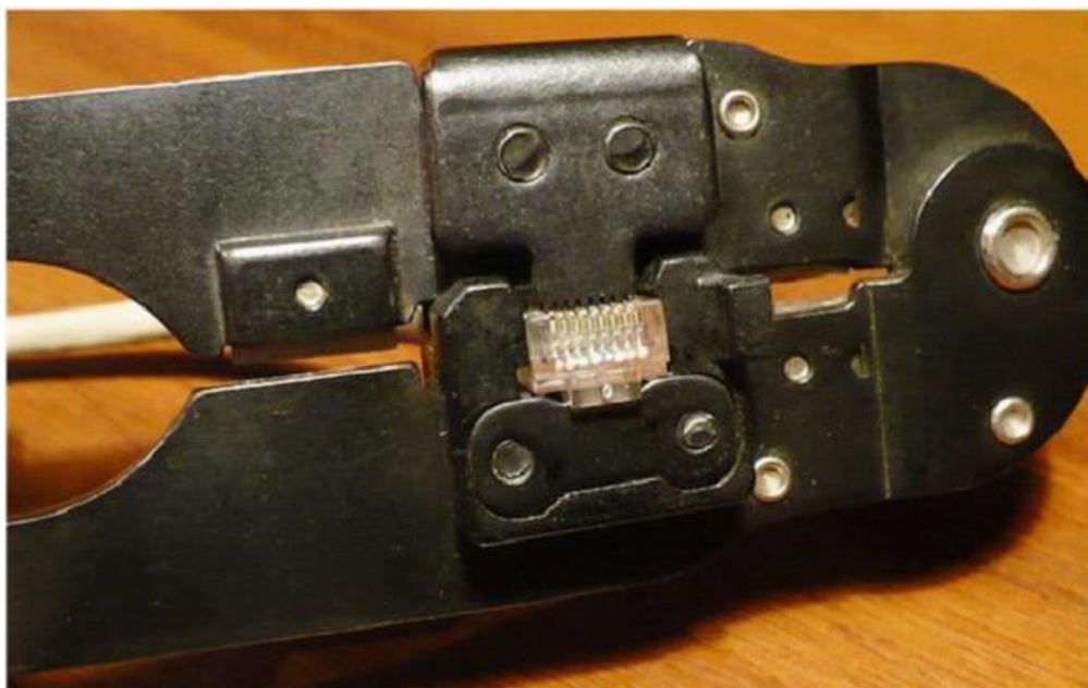
Рисунок 12.5 Обжим вилки RJ-45 на кабеле
