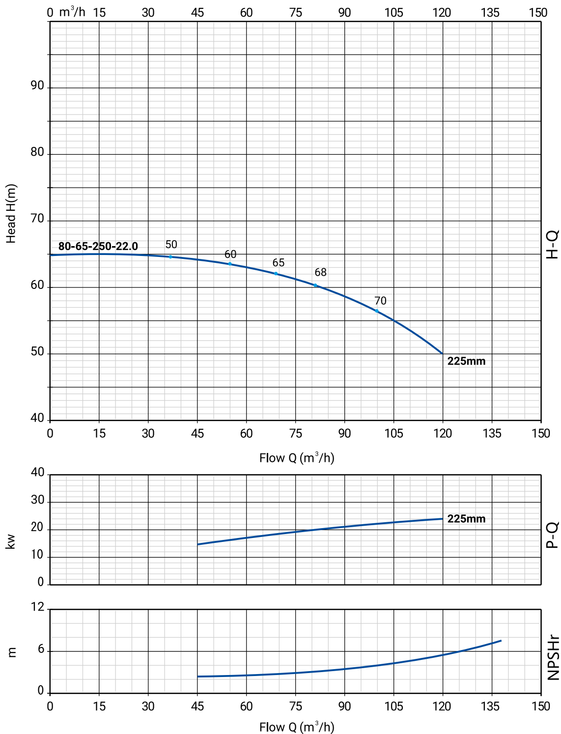
Рис.4. Пример графиков напор-расход, мощность, КПД, NPSH
