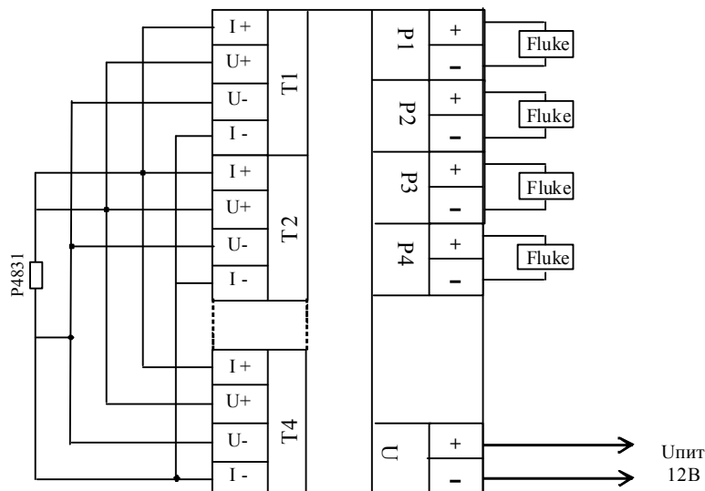
Схема подключения ТМК-Н130 к приборам и оборудованию при калибровке
